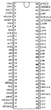
900 mil DIL 64 PIN
